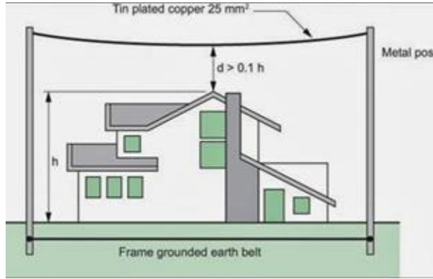
Figure 10 ഇടിമിന്നൽ സുരക്ഷാസംവിധാനം
