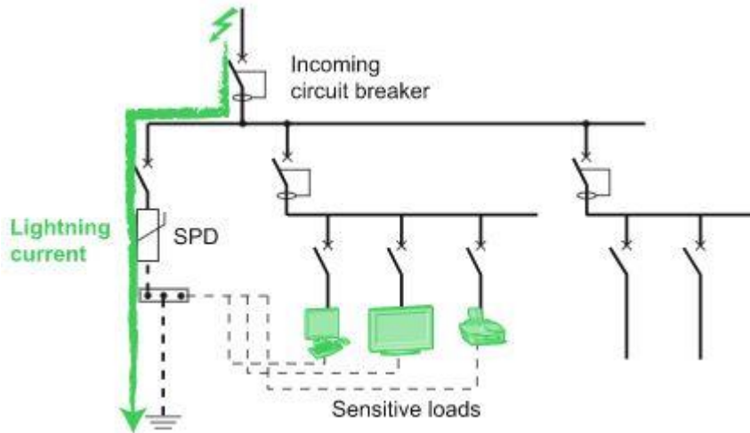
Figure 13 സർജ്ജ് സംരക്ഷണ ഉപകരണം
