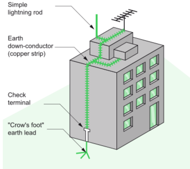
Figure 9 ഇടിമിന്നൽ സുരക്ഷാസംവിധാനം
